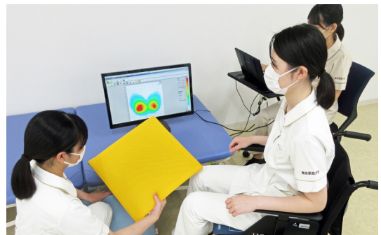
体圧分布センサーを用いた車椅子用クッションの性能評価
