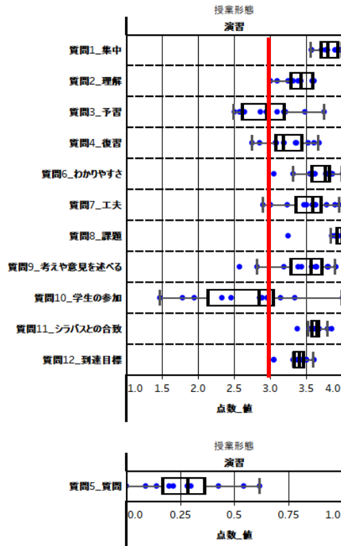
〈度数分布と平均値〉
