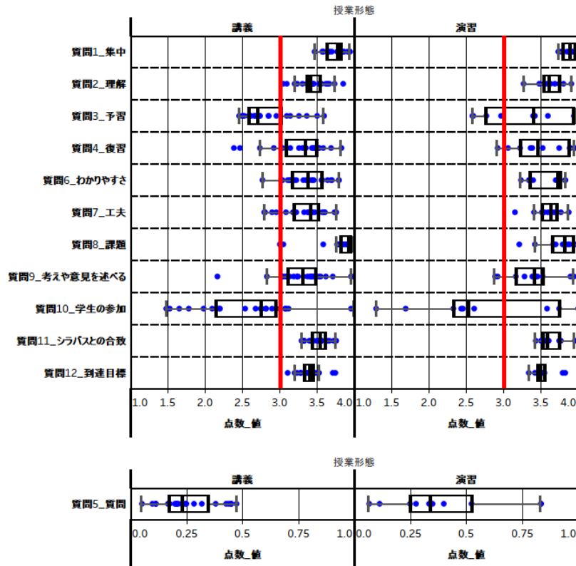
〈度数分布と平均値〉
